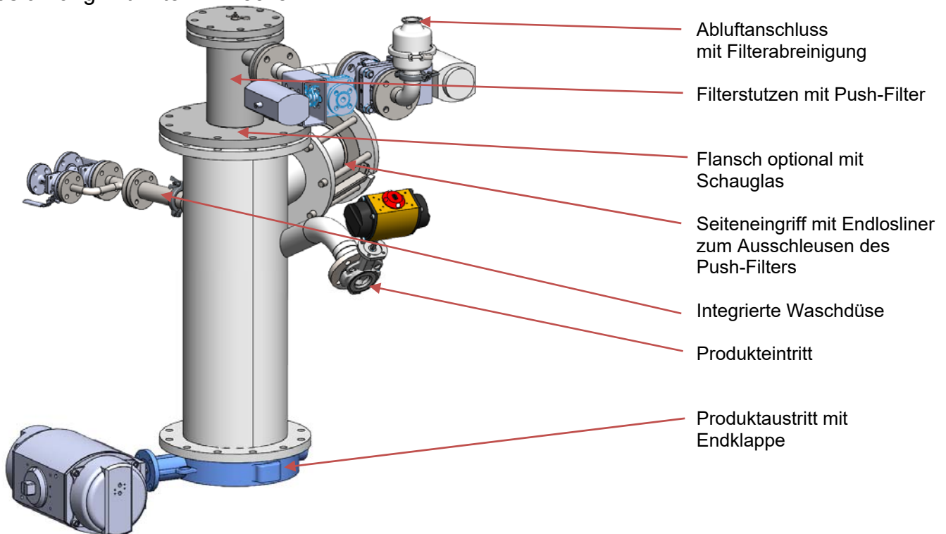
Ausführung mit Filter im Deckel
