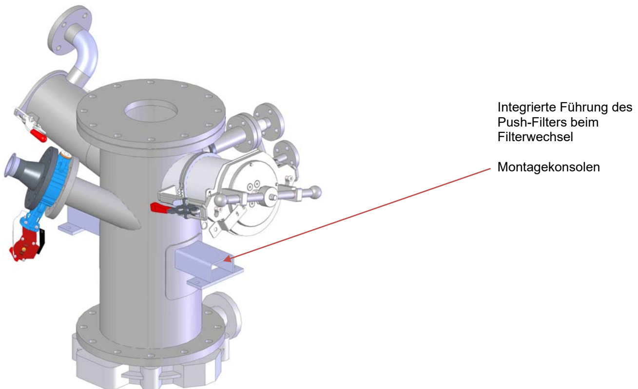
Ausführung mit Filter seitlich
